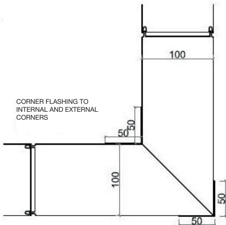
MITRED CORNER
